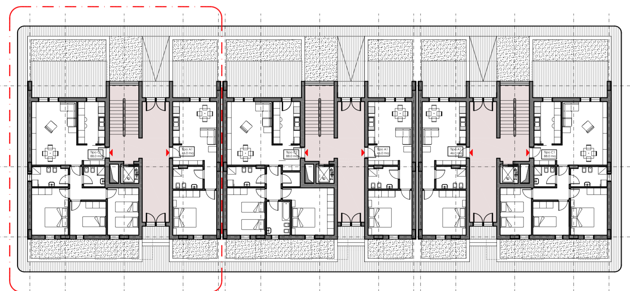
ESEMPLIFICATIVO PIANO TERRA edifici su comparto R1, R2, R4 - scala 1:200
