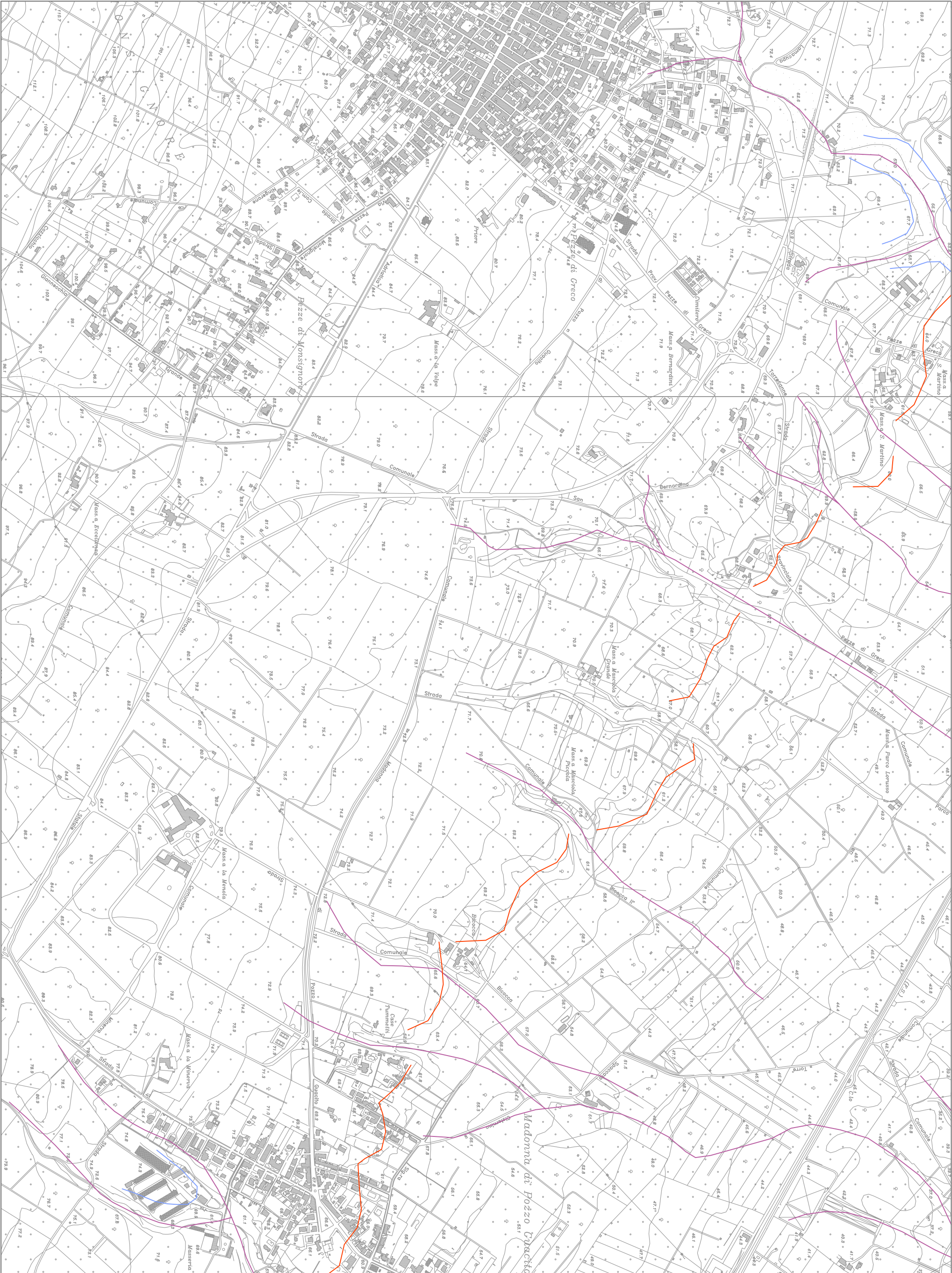
4-4 ATD geomorfologici
