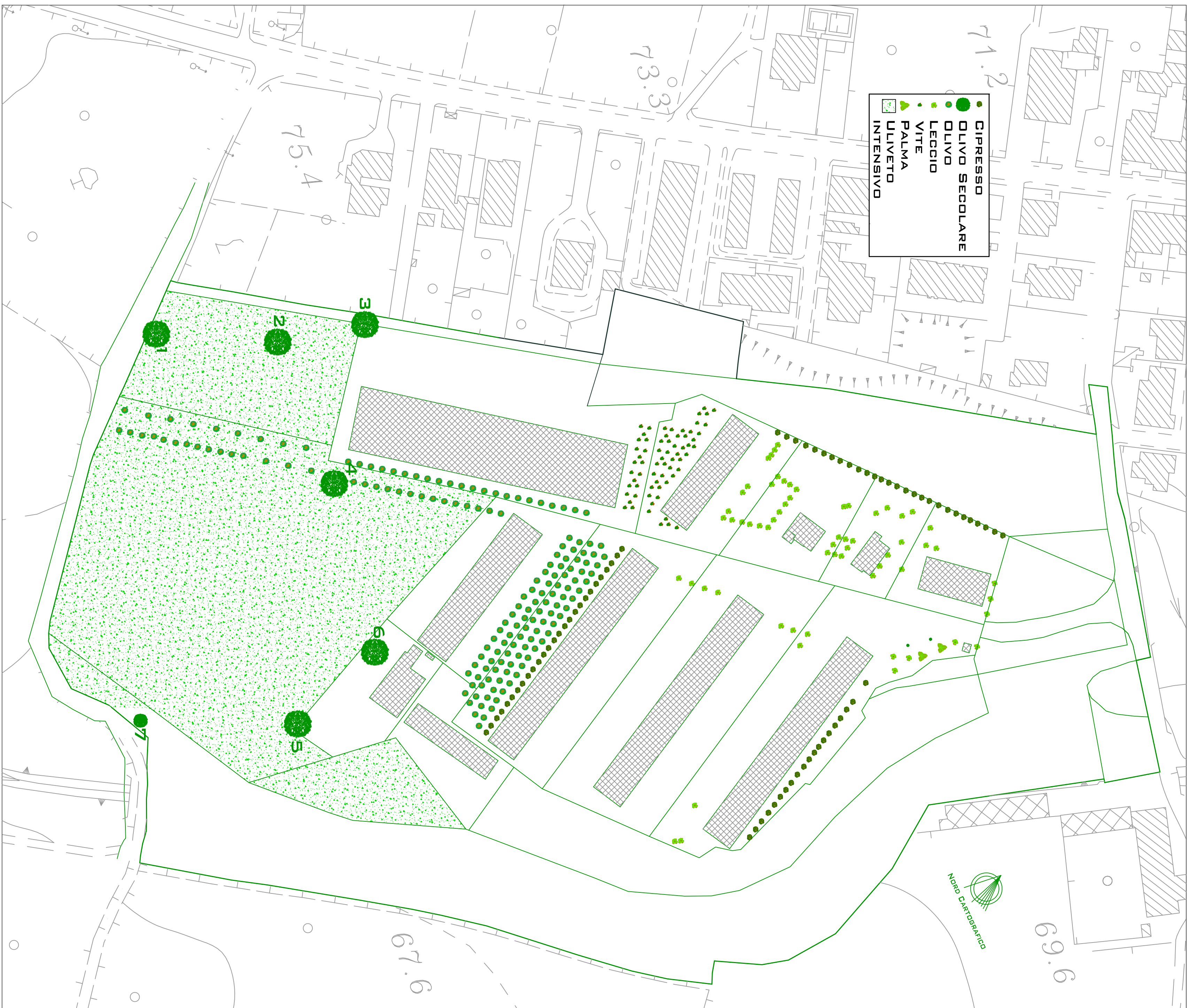
RILIEVO ALBERATURE ESISTENTI - SCALA 1:1000
