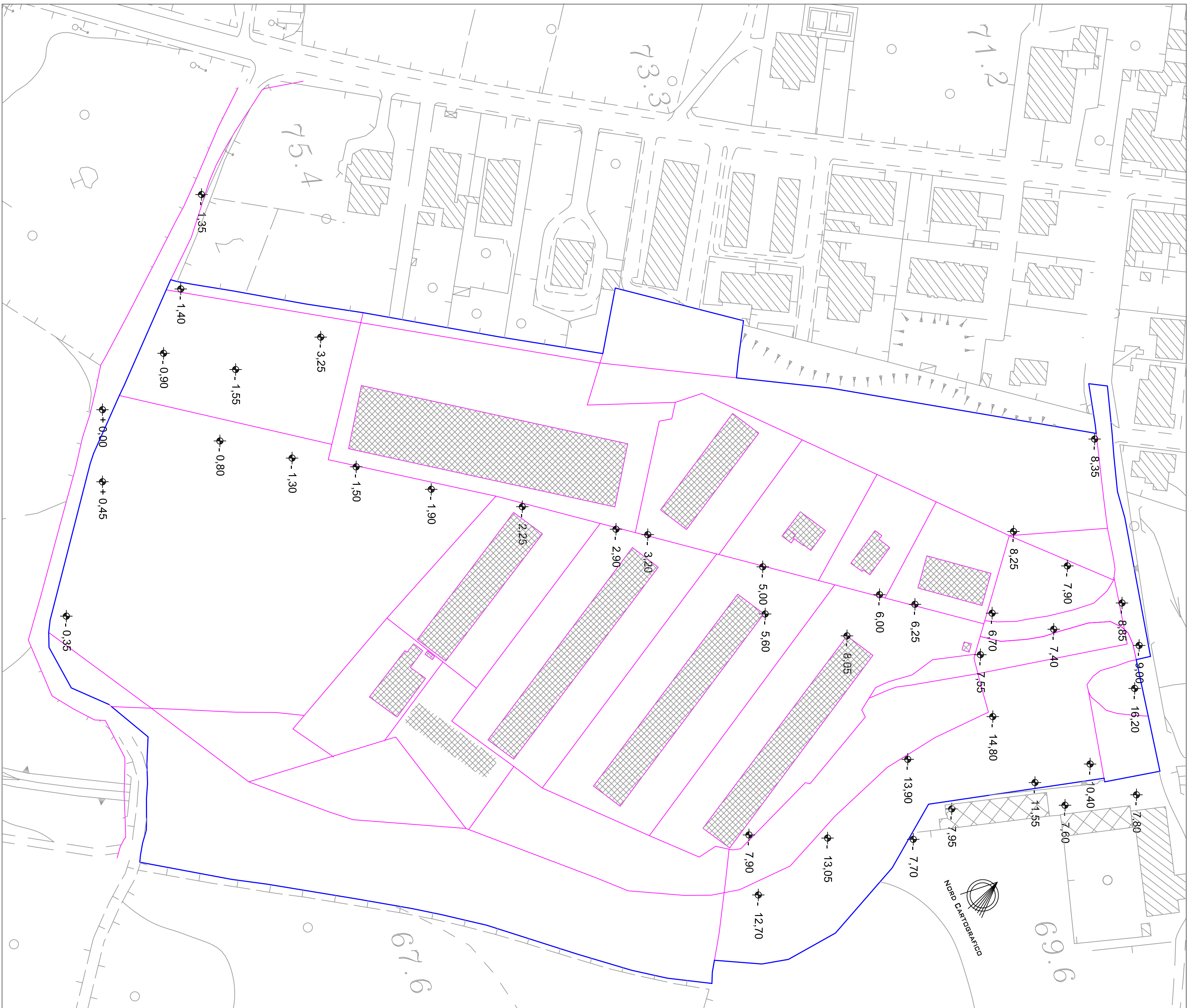
PIANO QUOTATO DEL SITO - SCALA 1:1000
