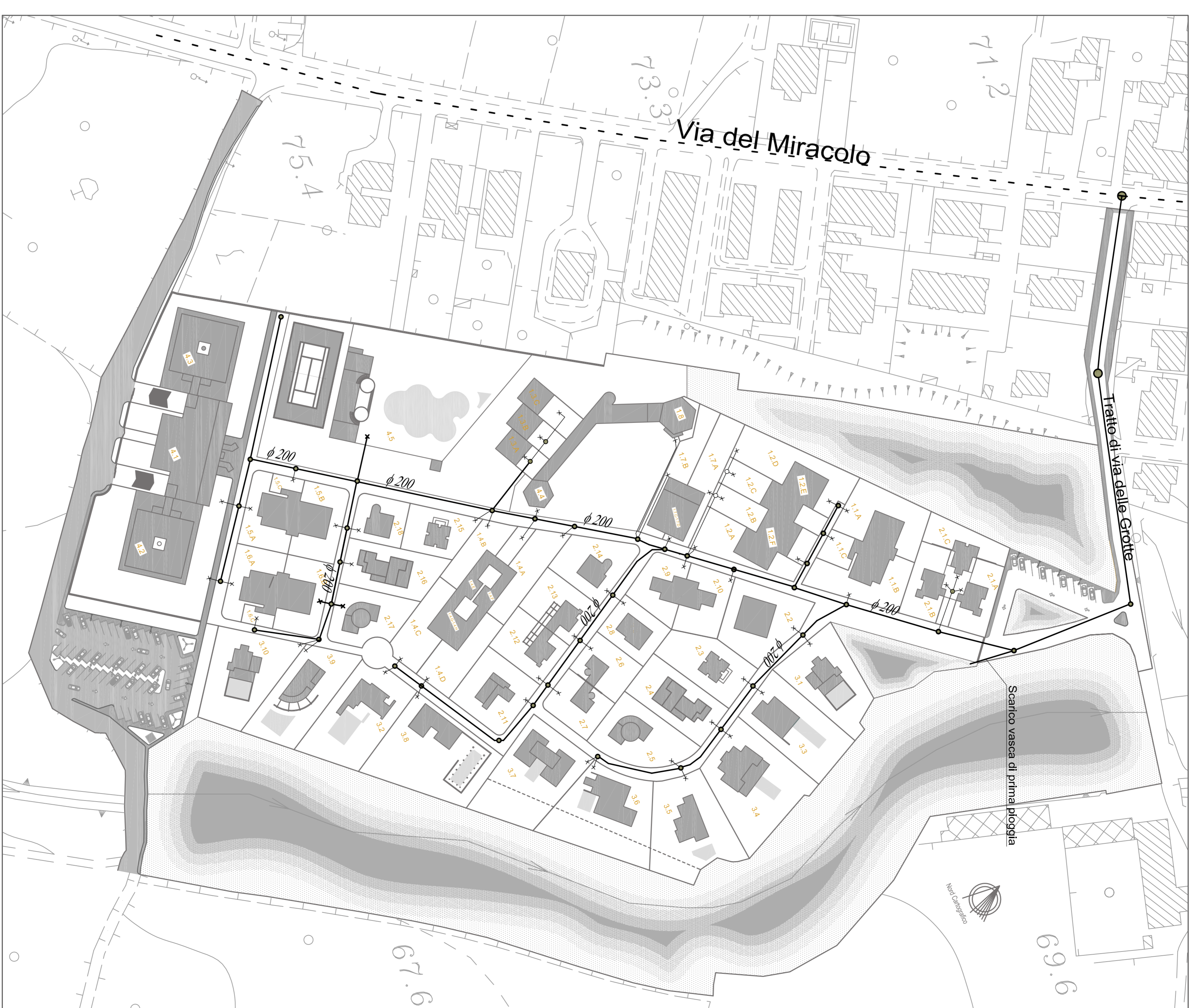
URBANIZZAZIONI DI PROGETTO: RETE FOGNARIA - SCALA 1:1000
