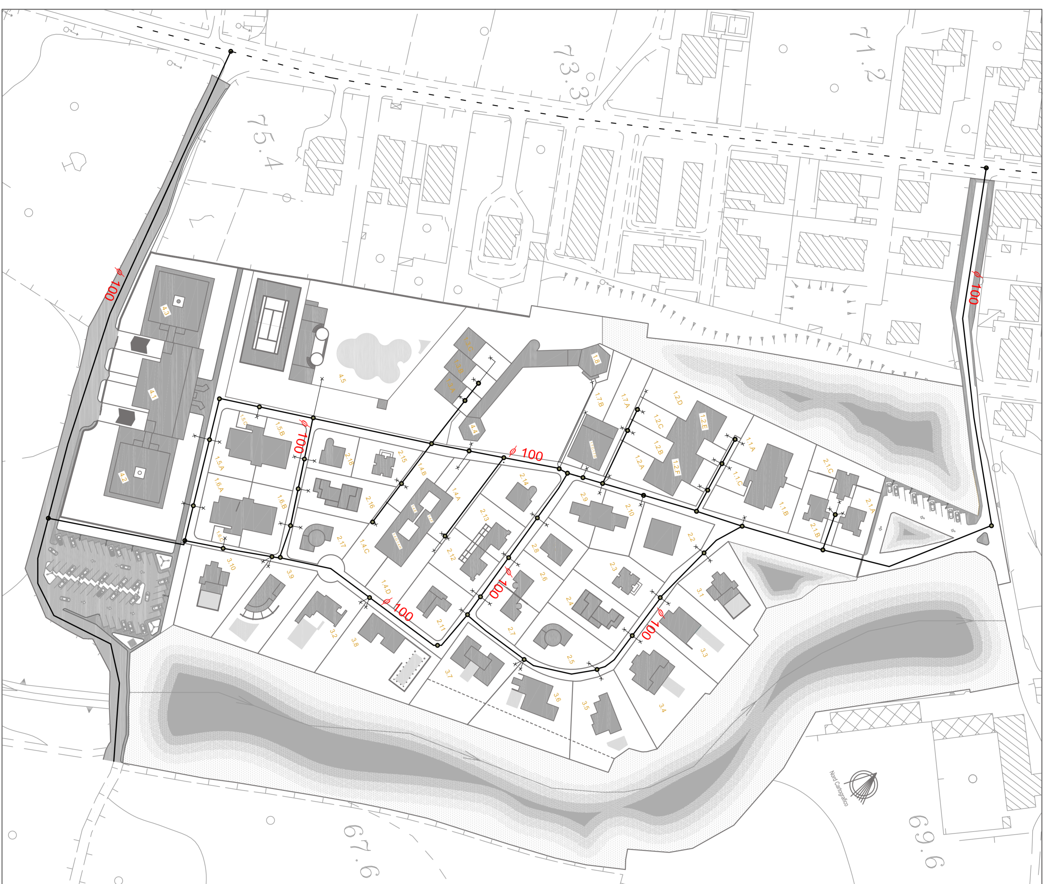
URBANIZZAZIONI DI PROGETTO: RETE IDRICA - SCALA 1:1000
